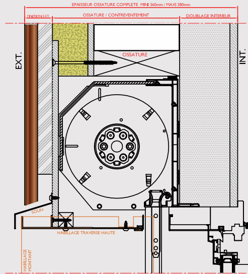
BLOC VOLET ROULANT DEMI-LINTEAU
