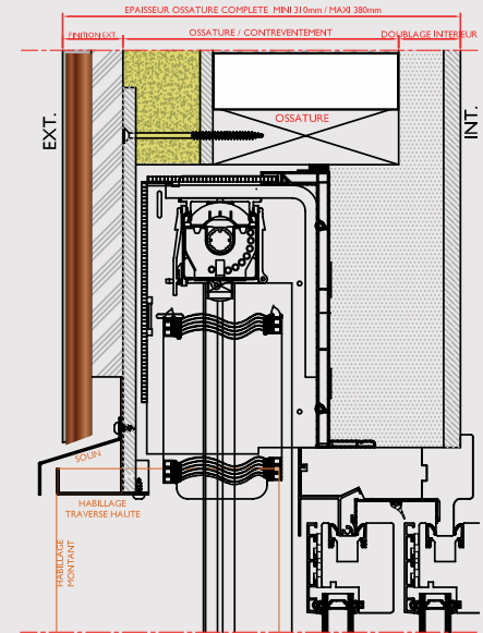
BLOC BRISE SOLEIL ORIENTABLE DEMI-LINTEAU
