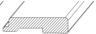
Moulure enrobée Pin ou Chêne pour recouvrement total de 80mm
