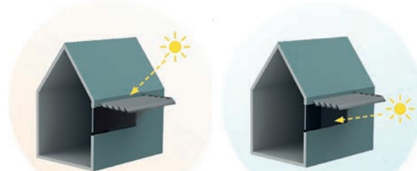
L'incidence en fonction des saisons du rayonnement solaire : à gauche, l'été et à droite, l'hiver. © Bluetek
